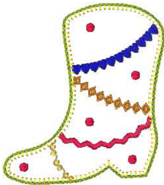
Ee220_03.art60
