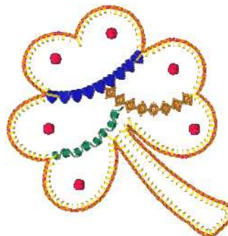
Ee220_06.art60
