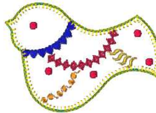
Ee220_02.art60
